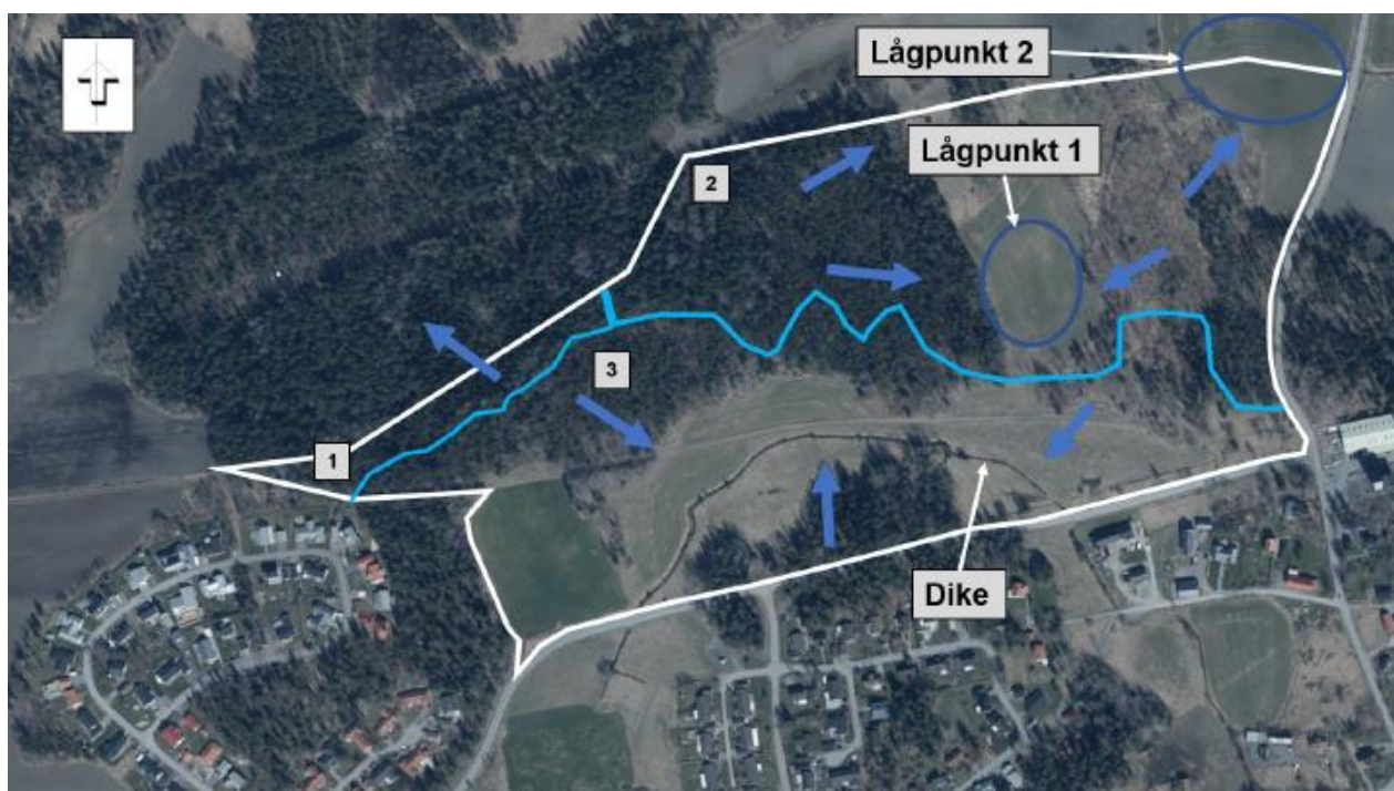
Figur 18: Områdesbild med ytavrinning för dagvatten, pilarna motsvarar vattnets flödesriktning.
