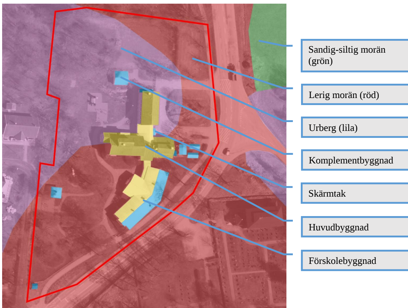
Figur 17: Plankarta som illustrerar dagvattenhantering för befintliga taktytor samt jordarter. Takytor med anslutning till kommunal dagvattenledning i gult. Takytor med utkastare på mark i blått.
