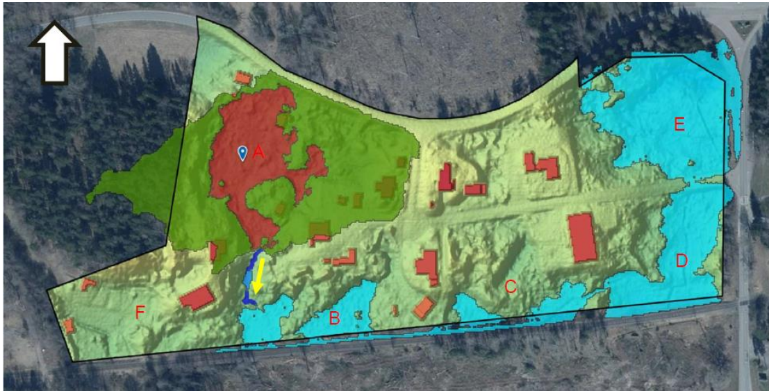
Figur 9. Avrinningsområde (grön) och utbredning (röd) av lågpunkt i område A. Gul pil visar flödesriktning vid brädning över vägen med vall-funktion mellan område A och B.
